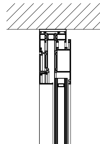
5 Detail 3 1 : 5
