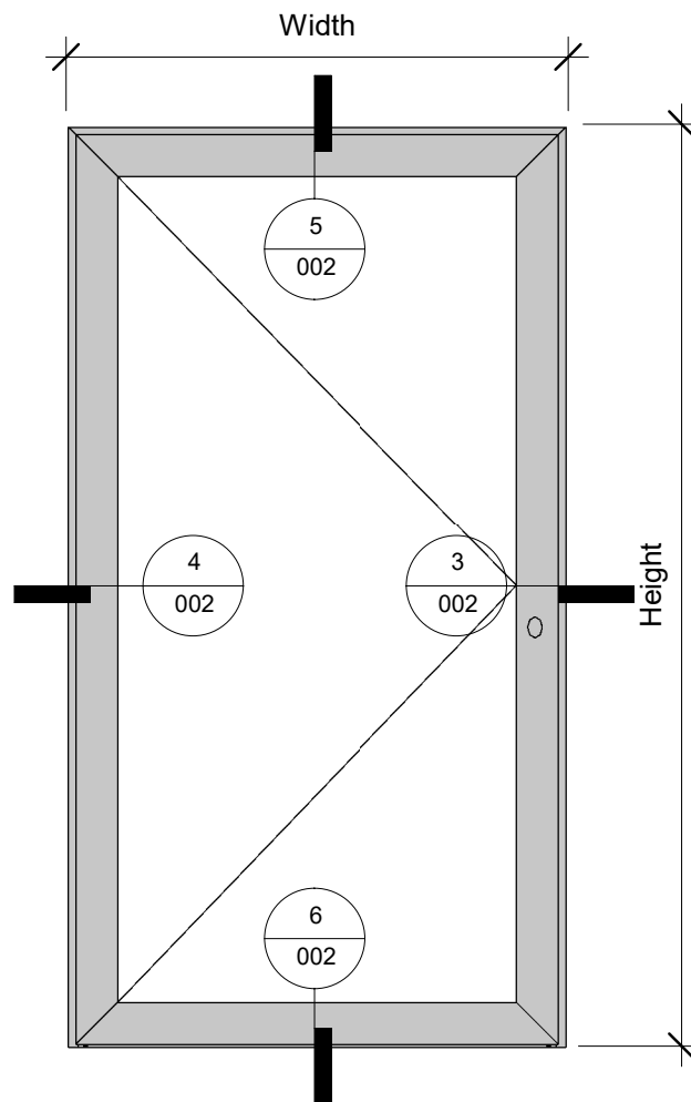
2 Elevation Back 1 : 20
