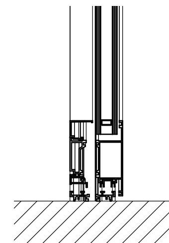
6 Detail 4 1 : 5
