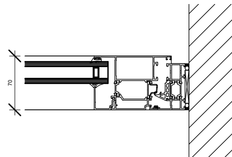
4 Detail 2 1 : 5
